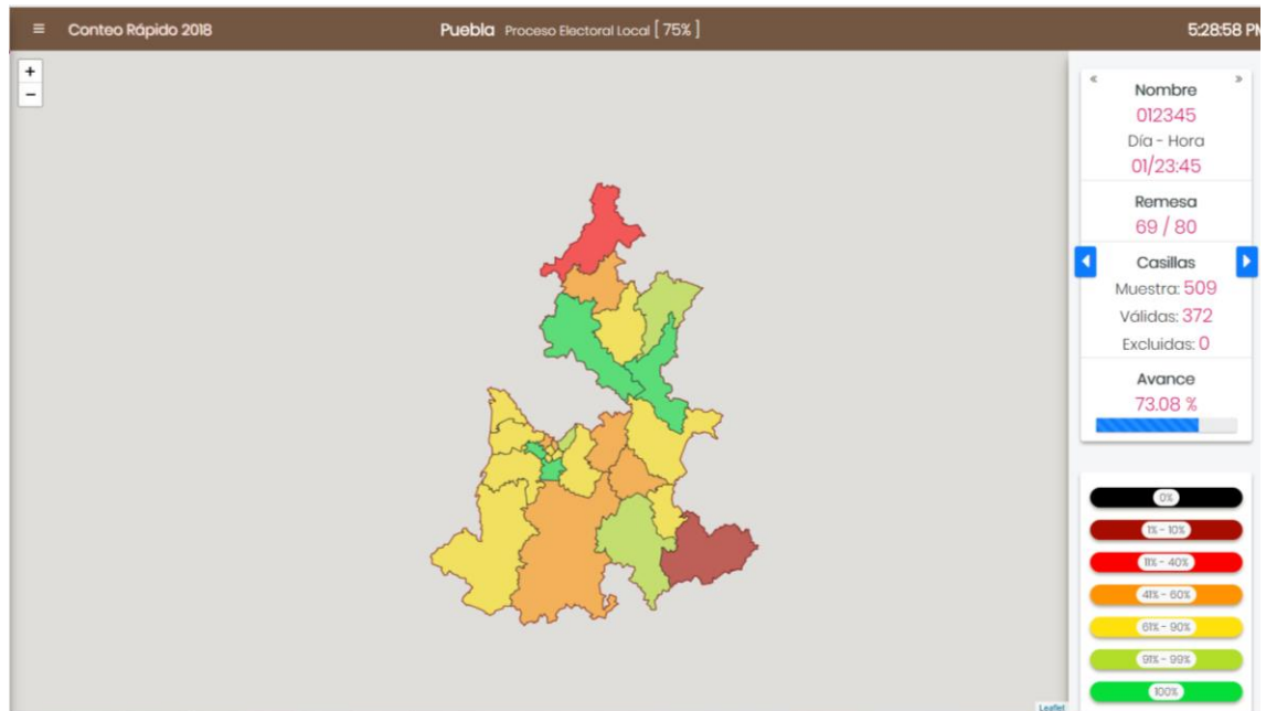
Conteo Rápido de Puebla. Cobertura geográfica de la muestra por estrato
